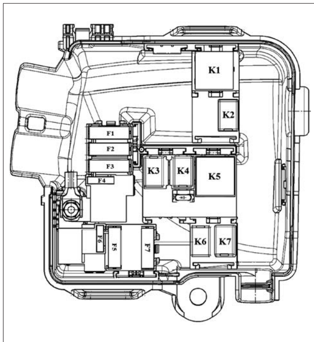
Рис. 2. Блок предохранителей и реле моторного отсека (ДВС 11189)
