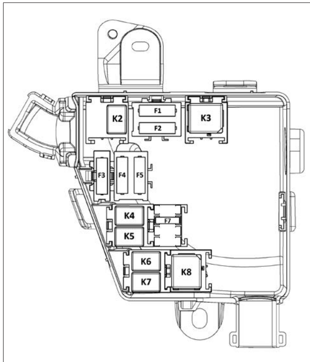
Рис. 3. Блок предохранителей и реле моторного отсека (ДВцС К4М)
