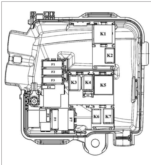
Рис. 2. Блок предохранителей и реле моторного отсека (DVS 11189)
