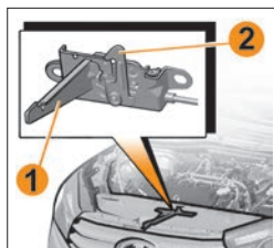
Рис. 2. Замок безопасности капота
